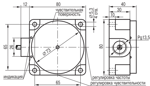
Габаритный чертеж
