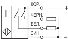
Схема подключения активной нагрузки
